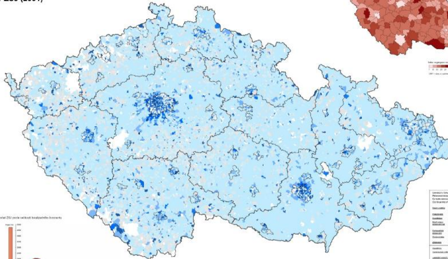
Lokalizační kvocient osob nad 15 let s VŠ vzděláním
